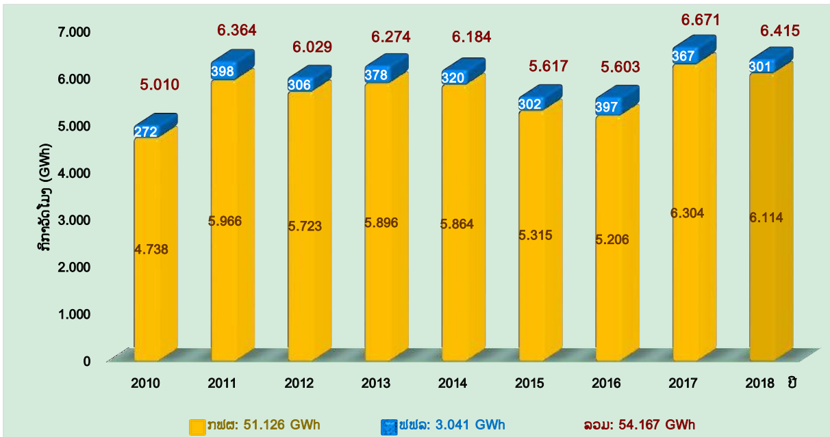
ພະລັງງານໄຟຟ້າຂາຍໃຫ້ ກຟຜ ແລະ ຟຟລ (ແຕ່ປີ 2010 ຫາ 2018)
